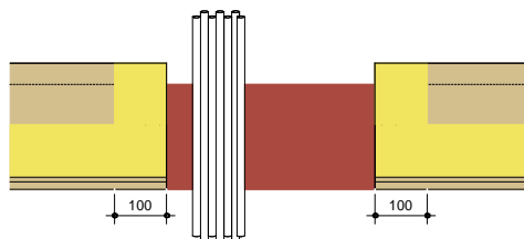
Exécution des joints Exemple EI 90
