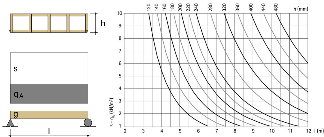
Figure 3: Toiture, exemple d'aptitude à l'emploi pour une déformation w = l / 300 ( t_i = 31 \text{ mm} , t_{ij} = 31 \text{ mm} , d = 31 \text{ mm} )
