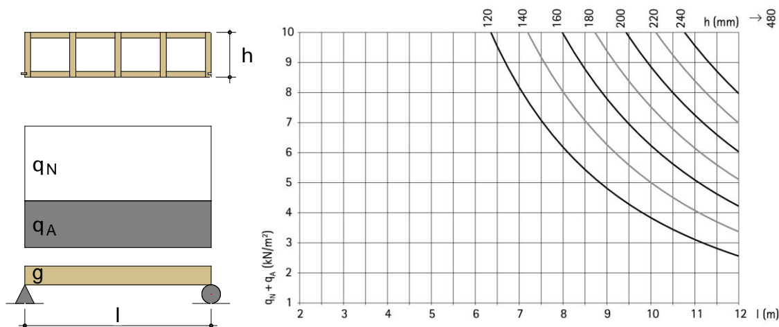
Figure 1: Exemple de capacité porteuse, flexion et cisaillement ( t_i = 31 mm, t_{iii} = 31 mm, d = 31 mm)
