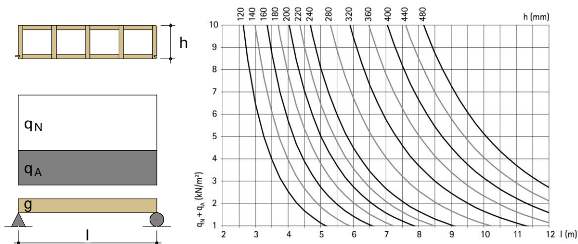
Figure 2: Plancher, exemple d'aptitude à l'emploi pour une déformation w = l / 600 ( t_i = 31 \text{ mm} , t_{ij} = 31 \text{ mm} , d = 31 \text{ mm} )
